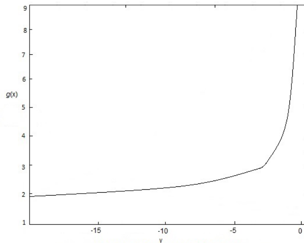
Figura 5. Función convexificada g(y) con \rho=2
