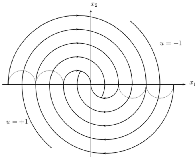
Figura 17. Trayectorias extremales para el oscilador lineal actuado.
