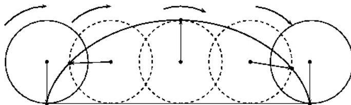
Figura 3. Cicloide: lugar geométrico de un punto fijo en un círculo que rueda sin resbalar sobre una recta.
