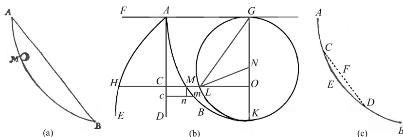
Figura 2. (a) El problema de la braquistócrona, (b) La solución de JOHANN BERNOULLI, (c) La solución de JACOB BERNOULLI.
