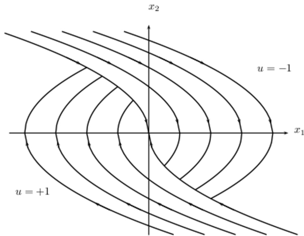
Figura 16. Trayectorias óptimas con un punto de conmutación.
