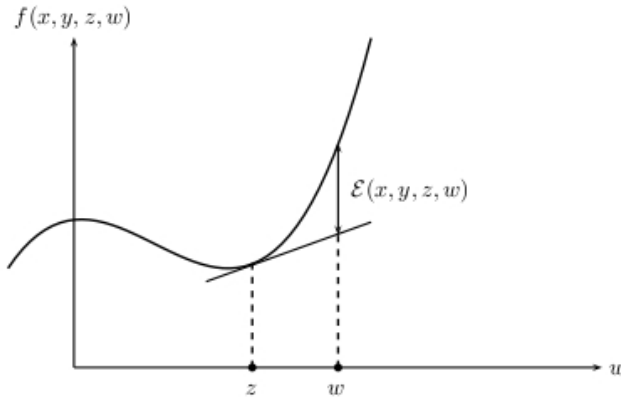
Figura 8. Interpretación geométrica de la función exceso de Weierstrass.
