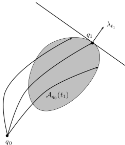
Figura 15. Hiperplano de soporte y covector normal al conjunto alcanzable.
