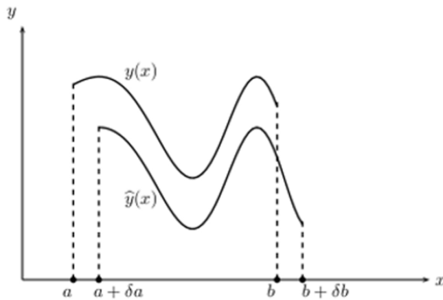
Figura 6. Dos curvas cercanas.
