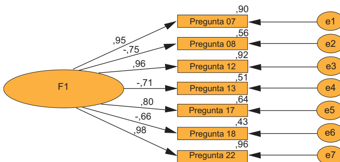
Figura 1. Modelo de un factor, M1F, e  tems que lo constituyen
