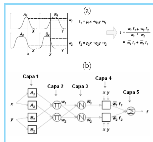
Figura 4. Arquitectura ANFIS para dos semáforos. a) Relaciones difusas. b) Equivalente ANFIS
