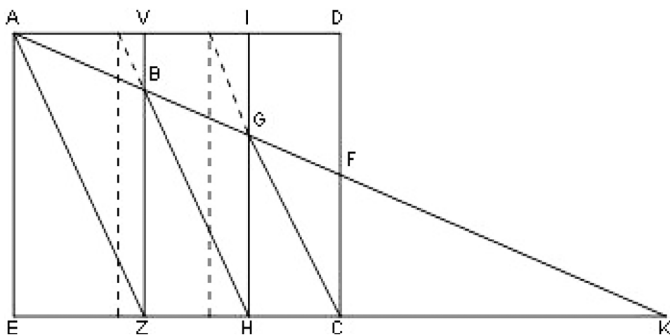
Figura 2. Mesolabio con los puntos alineados. 11
